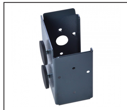
Bedienpulthalter magnetisch
