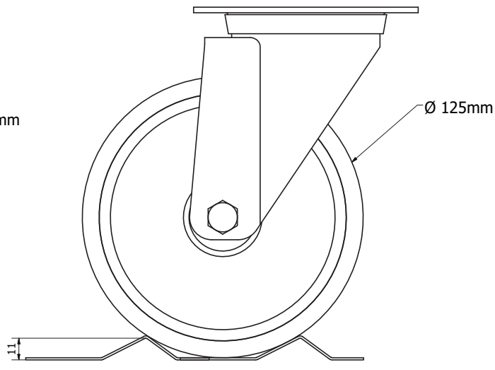
PARKBUCHT 11mm
